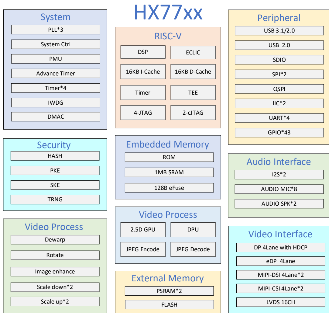
图 1-1 HX77xx 架构框图
